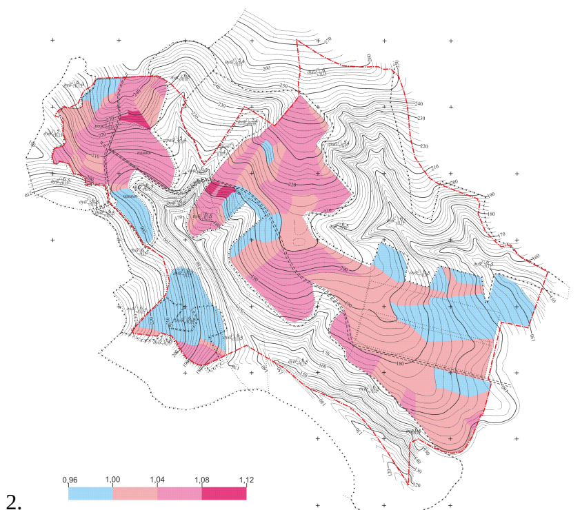
Рис. Карта распределения суммарной коротковолновой радиации на склоны в х. Пуляковском (опытное поле ВНИИВиВ) – 1 и в Анапе (ЗАО «Скалистый берег») – 2
